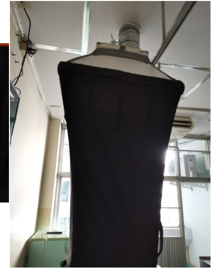
รูปวัดอัตราการไหลเชิงปริมาตรบริเวณช่องจ่ายอากาศเข้าห้อง
