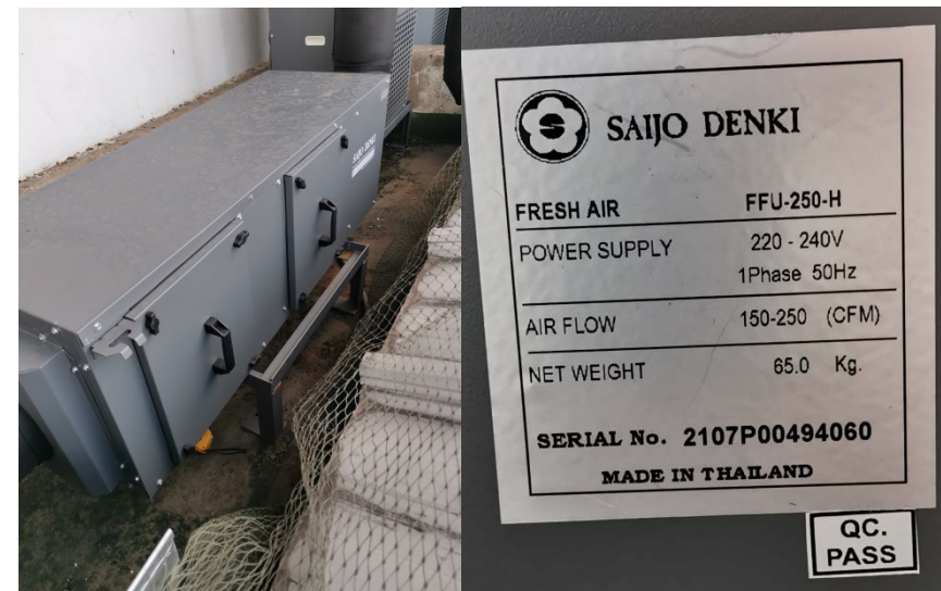
รูปแสดงชุดเครื่องระบายลมออกจากห้อง
